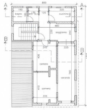
PIANTA PIANO TERZO SOTTOTETTO
